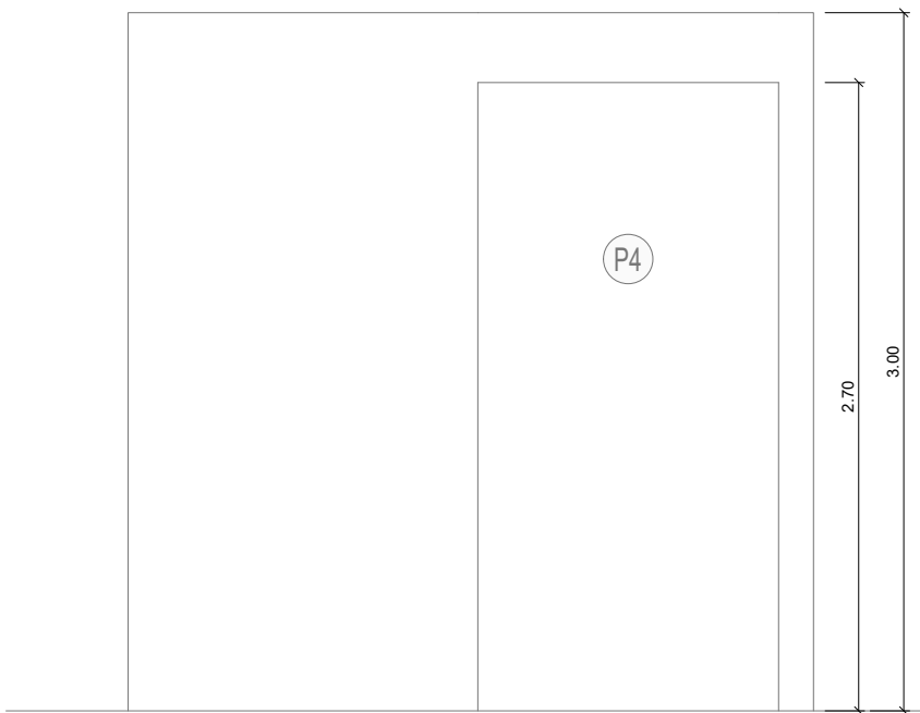
VISTA
